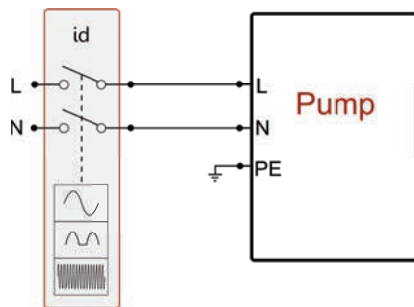
Фигура 11 – bis пример на инсталация
