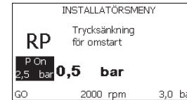
Fig. 17: Inställning av tryck för omstart
