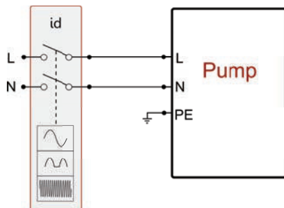
Obr. 11 – bis Příklad instalace
