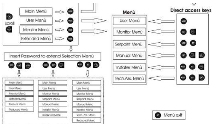
Afb. 14: Schema van toegangsmogelijkheden tot het menu
