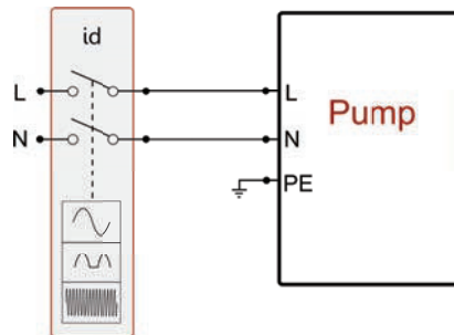
Kuva 11 - bis Esimerkki asennuksesta
