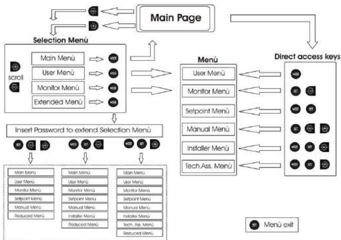
Kuva 14: Valikoiden avauskaavio
