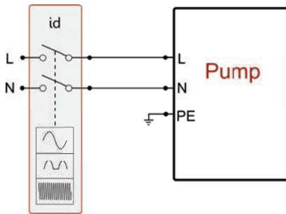
Figura 11 - exemplo de instalação
