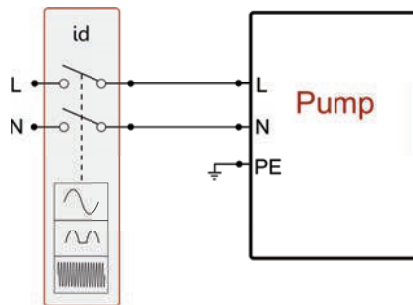
Рисунок 11 - bis Пример установки
