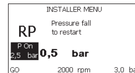
Kuva 17: Uudelleenkäynnistysarvo asetettu
