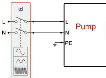
Afb. 11 - bis voorbeeld van de installatie
