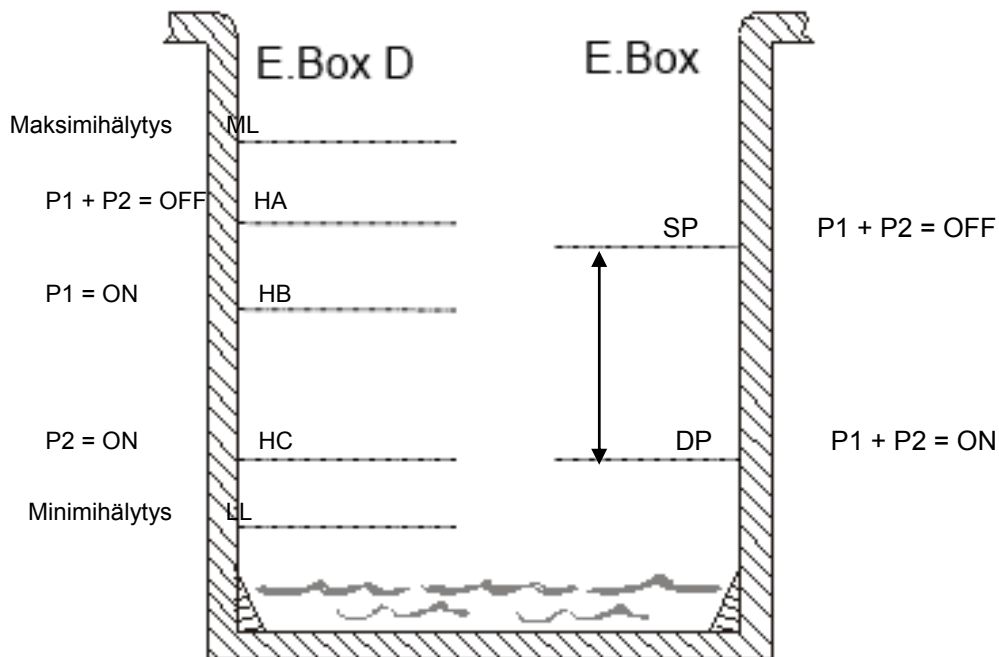
Kuva 30. Täyttö syvyyssanturilla
