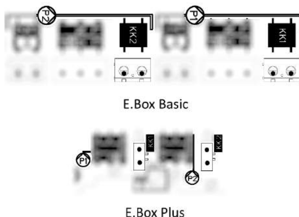
Εικόνα 9: Είσοδοι θερμικής προστασίας KK
