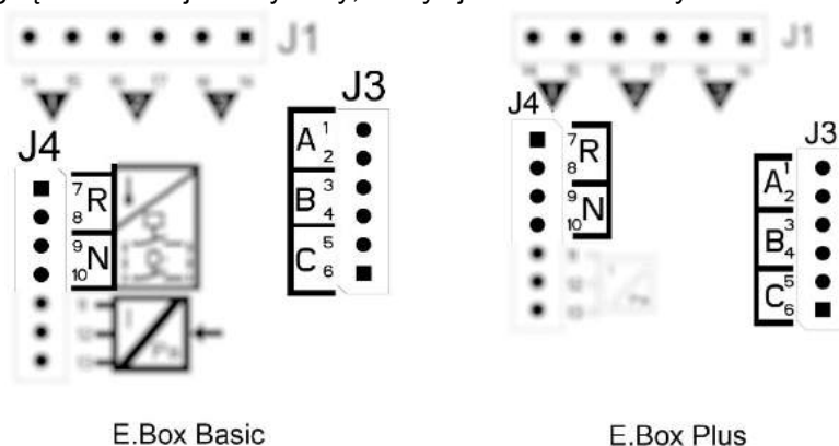
Rysunek 44: Wejścia
