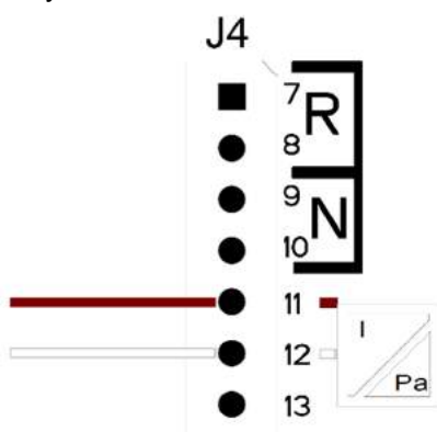
Схема 10: Подсоединение датчика давления 4..20mA
