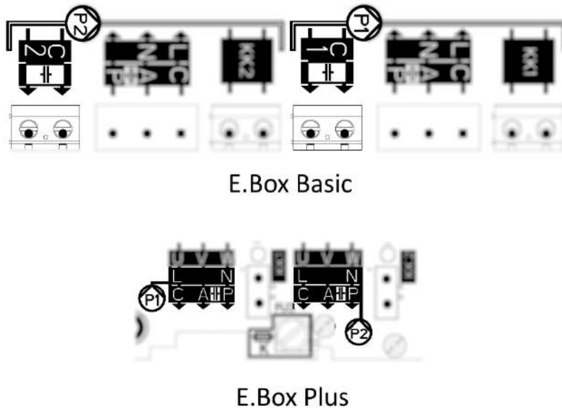
Figura 4: Conexión de los condensadores externos de las bombas
