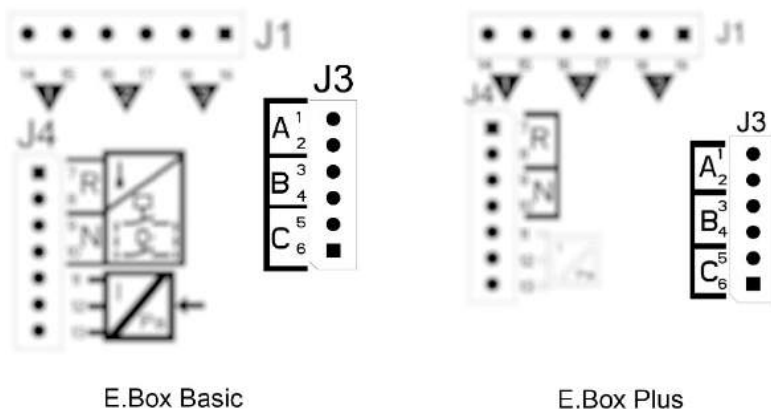
Figura 47: Borna presostați
