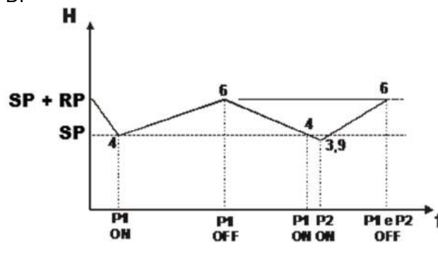
Figura 18: Reglare cu vas de expansiune > 100 litri
