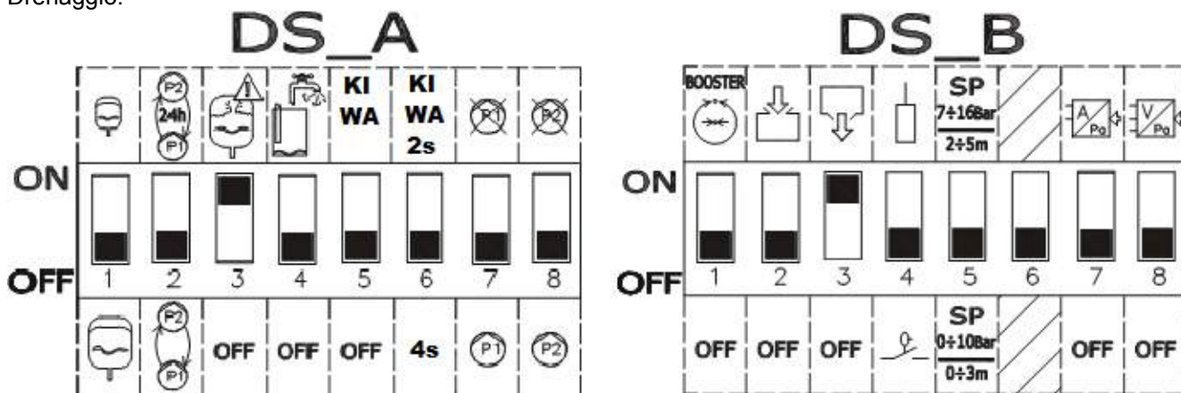
Figura 40: Impostazione dip switch Drenaggio
