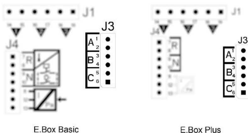
34.ábra: Bemenetek
