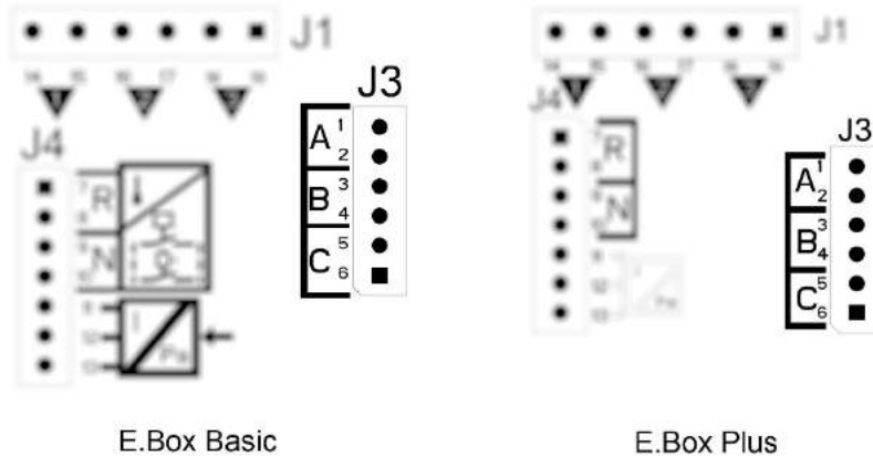
Εικόνα 22: Είσοδοι
