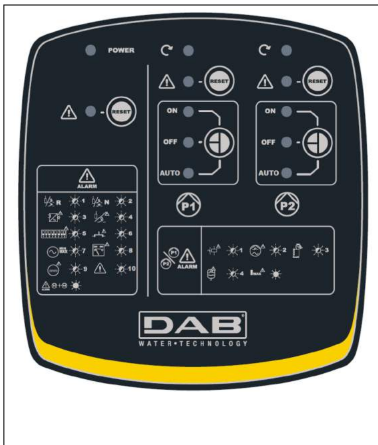
Figura 6: Etichetta display, presente solo nei modelli plus
