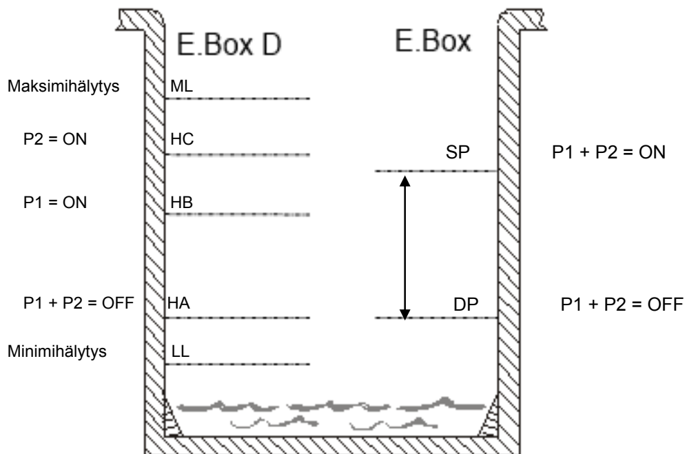
Kuva 43. Tyhjennys syvyyssanturilla
