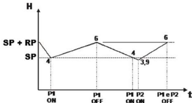
Rysunek 55: Regulacja z naczyniem zbiorczym > 100 litrów
