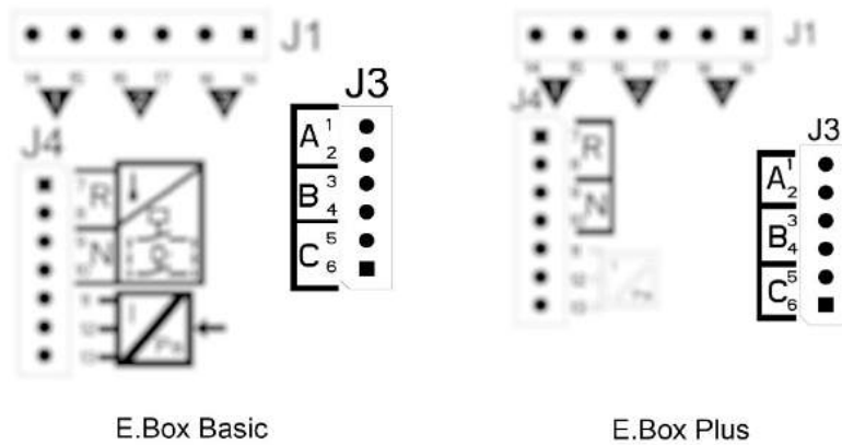
Схема 11: Клеммы для подключения реле давления
