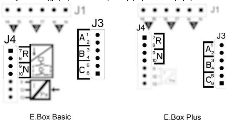
Εικόνα 44: Είσοδοι
