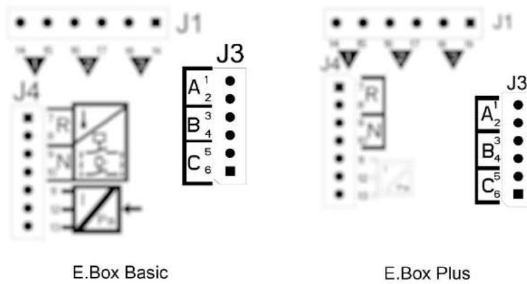
Figure 11 : Bornes pour le branchement des pressostats
