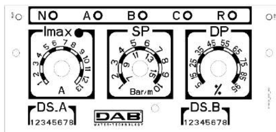
Εικόνα 29: Ρύθμιση ονομαστικής έντασης SP και DP
