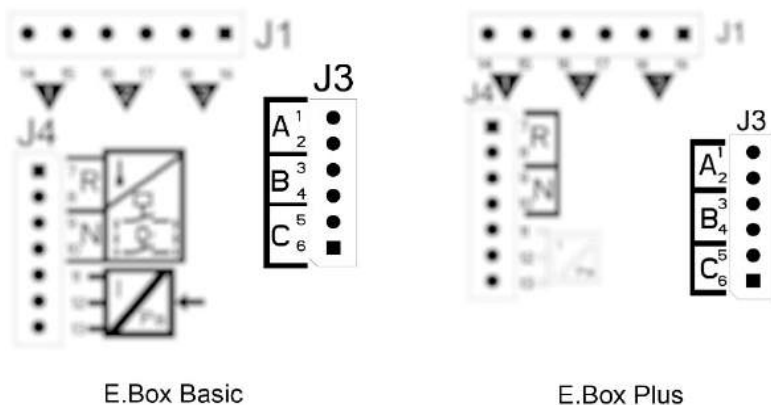
Afbeelding 47: Klemmenbord drukschakelaars
