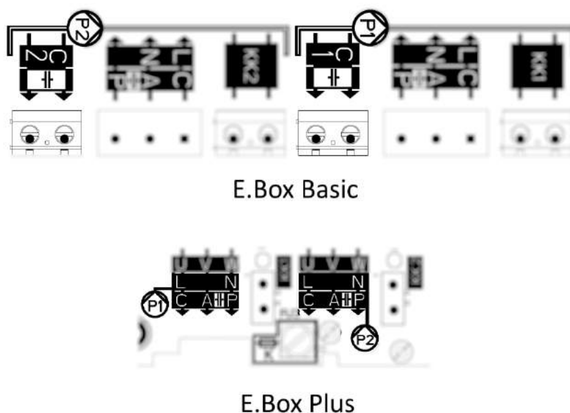
Схема 4: Соединение внешних конденсаторов насосов
