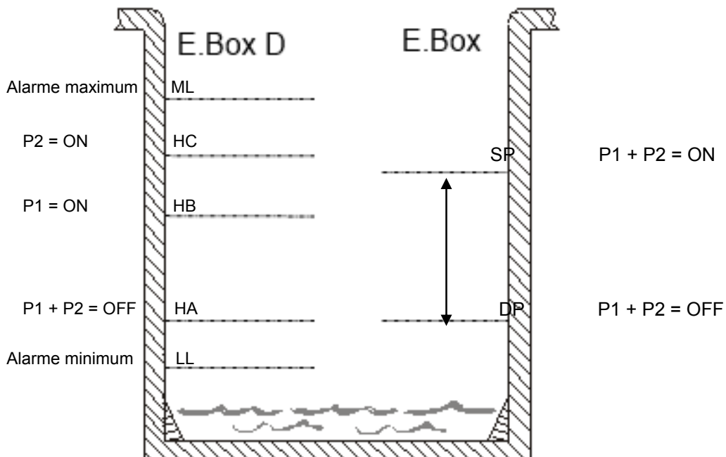
Figure 43 : Drainage avec capteur de profondeur
