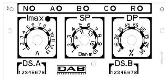
Abbildung 29: Einstellung des Nennstroms SP und DP
