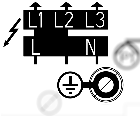
Kuva 5. Sähköverkon liitäntä.
