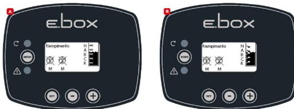
Figura 25: Starea sistemului în modalitate umplere, cu intrări de control plutitori sau sonde de nivel
