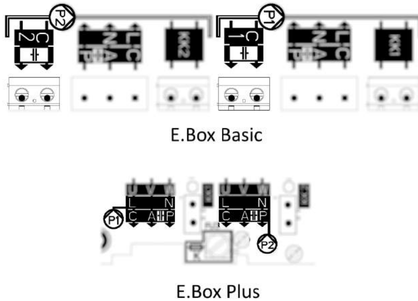
Figura 4: Collegamento condensatori esterni pompe
