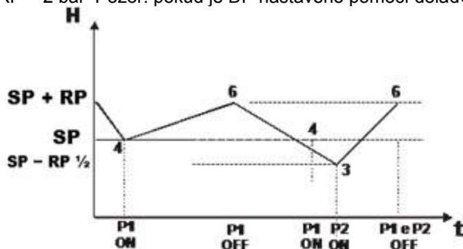
Obrázek 17: Regulace s expanzní nádobou < 100 litrů
