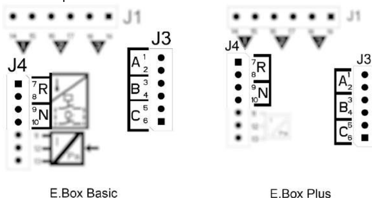
Figura 44: Entradas
