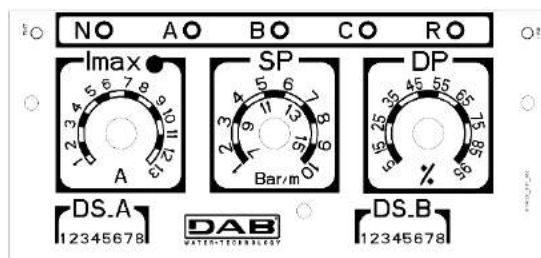
Figura 42: Reglare curent nominal SP și DP
