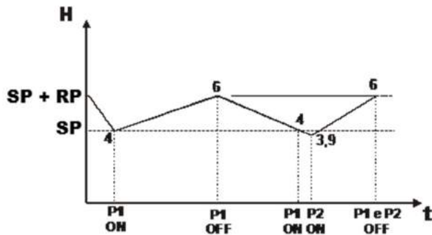
55.ábra: Szabályzás 100 liternél nagyobb táglási tartály esetén
