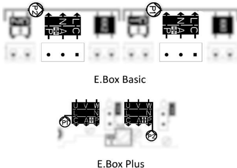
Figure 3 : Branchements électriques des pompes
