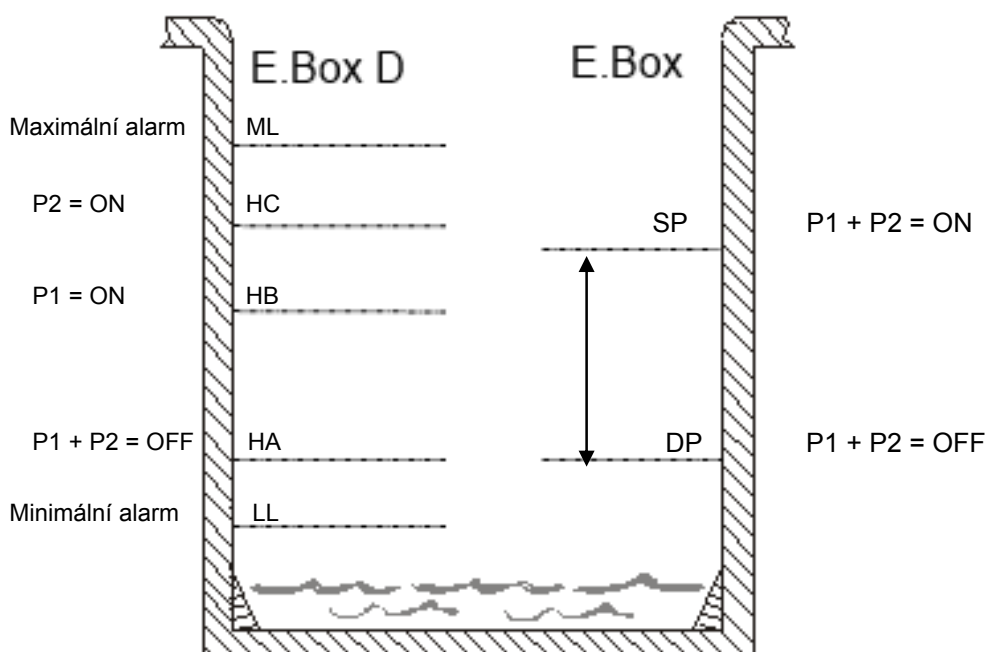
Obrázek 43: Vypouštění s hloukovým čidlem
