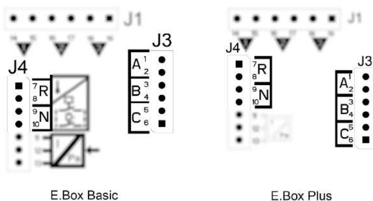
Figura 32: Pozitie intrări și alarme
