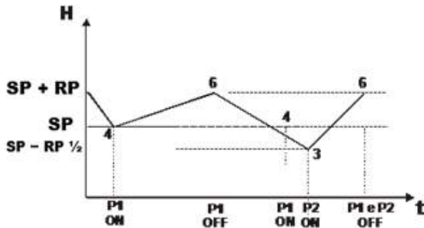
Rysunek 54: Regulacja z naczyniem zbiorczym < 100 litrów
