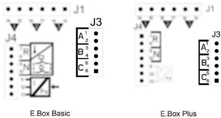
Kuva 11. Paineatkaisimien liittimet
