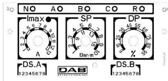
16. ábra: Az I_{max} , SP és DP beállítása
