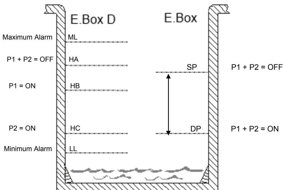
Rysunek 30: Napędzanie z czujnikiem głębokości
