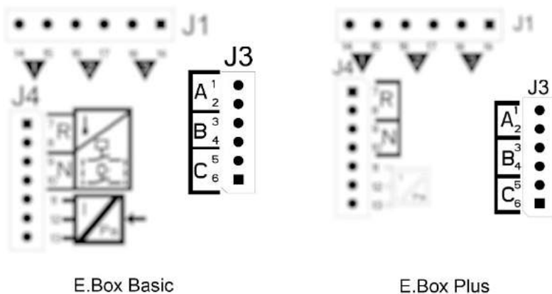
Kuva 47. Paineatkaisimien liitinalusta
