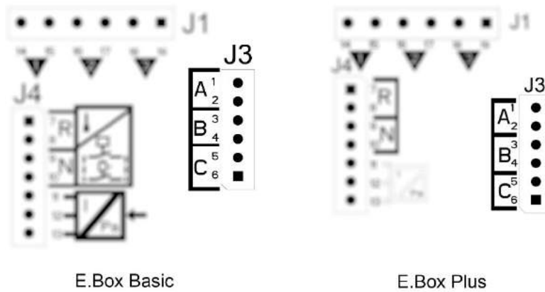
Figura 11: Borne pentru conectarea presostațiilor
