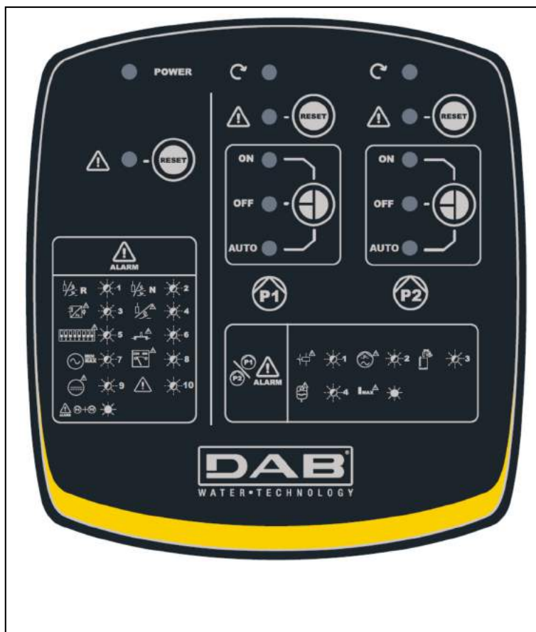
Kuva 7. Etupaneelin merkinnät
