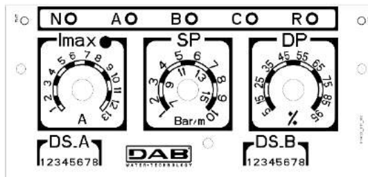
Afbeelding 42: Regeling nominale stroom SP en DP
