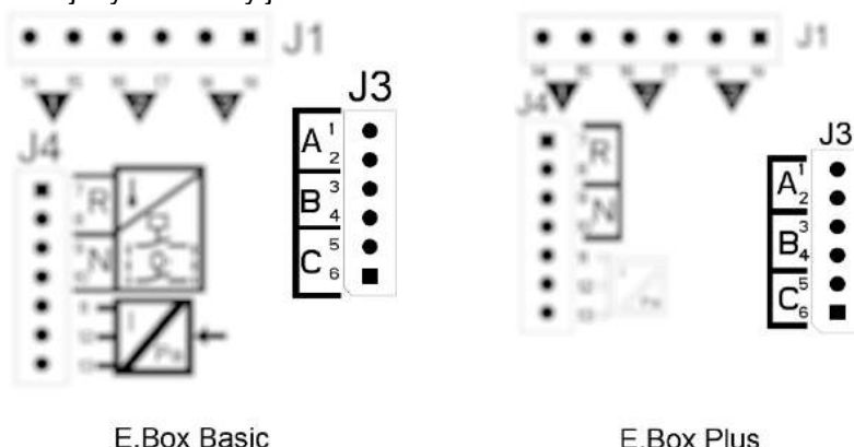
Obrázek 22: Vstupy
