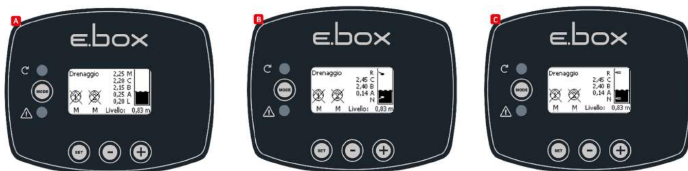
Схема 39: Состояние системы при конфигурациях: А только с датчиком глубины, В: датчик глубины и поплавки, С датчик глубины и зонды уровня.
