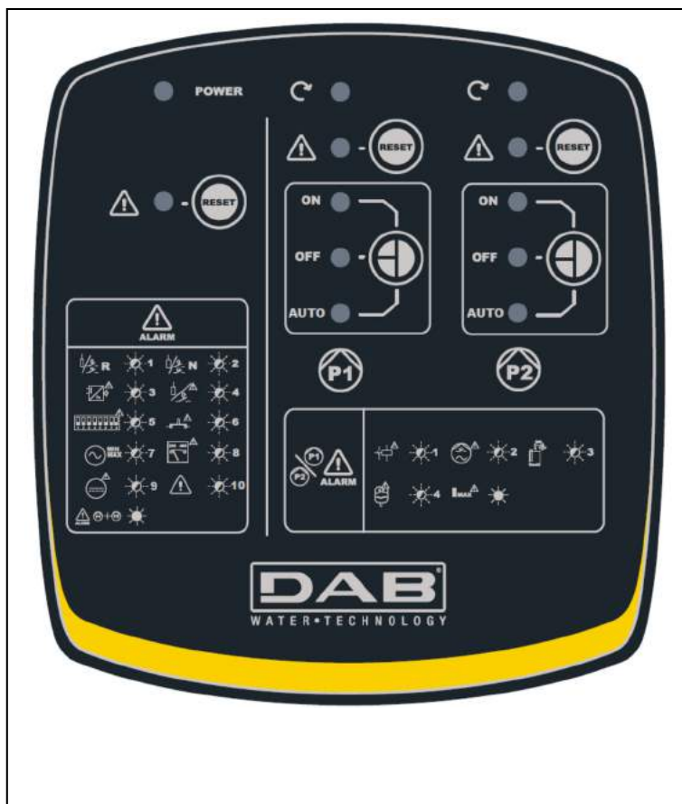
Figure 7 : Étiquette avant
