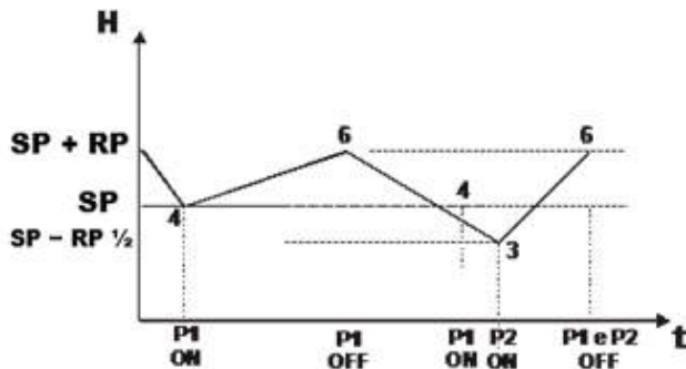
54.ábra: Szabályzás 100 liternél kisebb táglási tartály esetén
