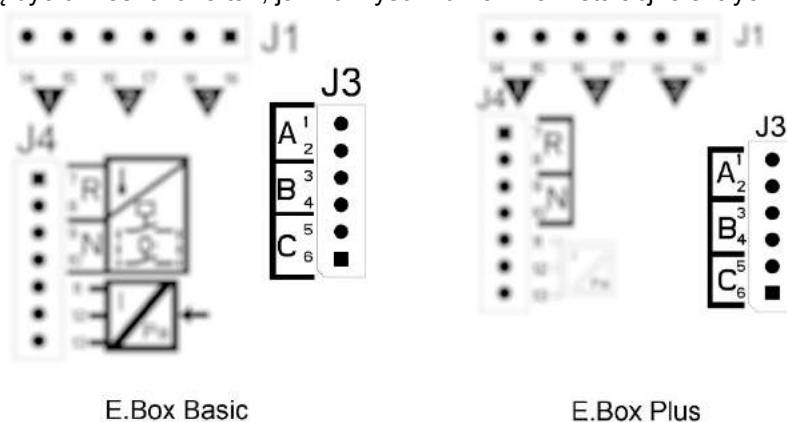
Rysunek 22: Wejścia
