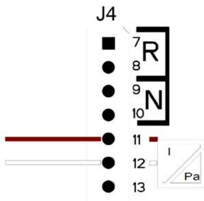
Схема 46: Подсоединение датчика давления 4..20mA
