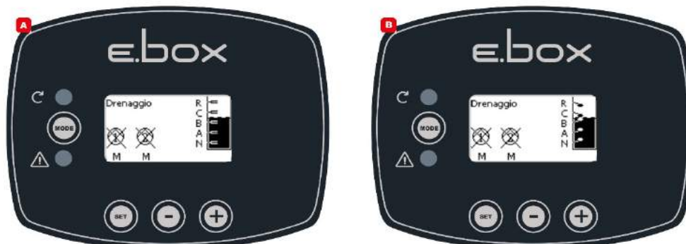
Abbildung 37: Status des Systems im Drainagemodus, A mit Standsonden. B mit Schwimmerschaltern
