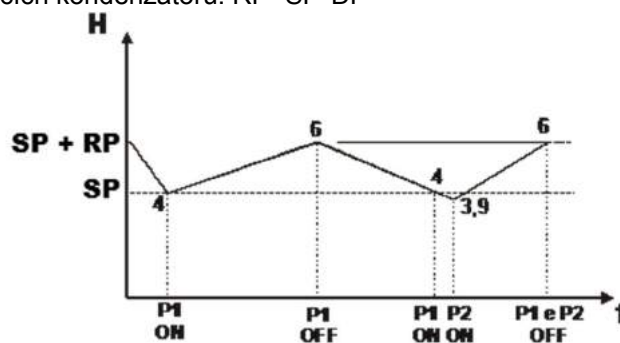
Obrázek 18: Regulace s expanzní nádobou > 100 litrů
