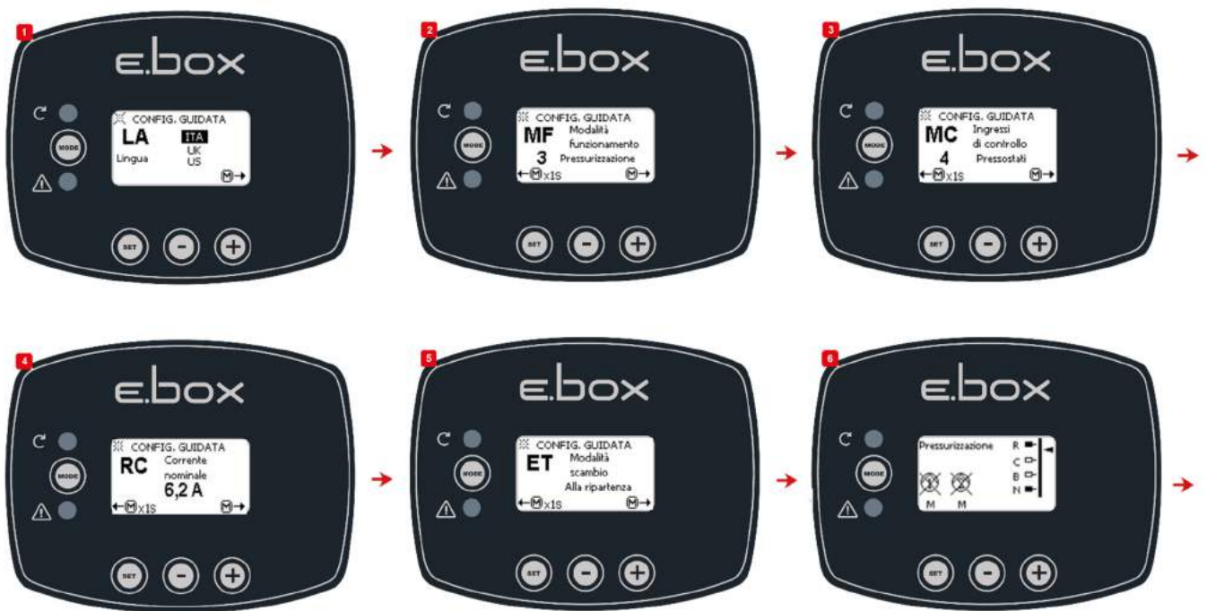
Obrázek 13: Nastavení s tlakovými spínači
