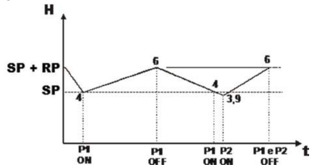
Figura 18: Regolazione con vaso di espansione > 100 litri
