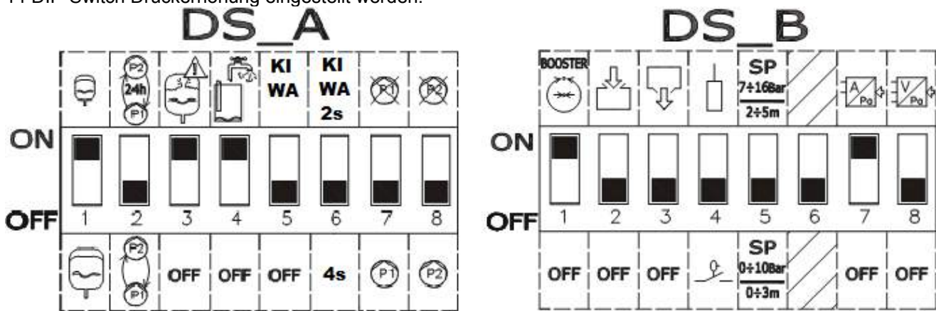
Abbildung 14: DIP-Switch Druckerhöhung
