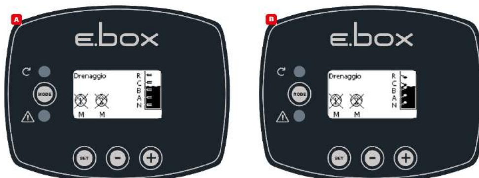
Rysunek 37: Stan układu w trybie drenażu, A z sondami poziomymi, B z pływakami
