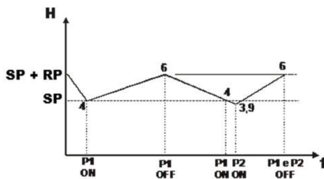
18.ábra: Szabályzás tágulási tartállyal mely>100liter
