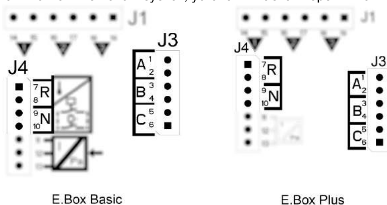
Схема 44: Вводы
