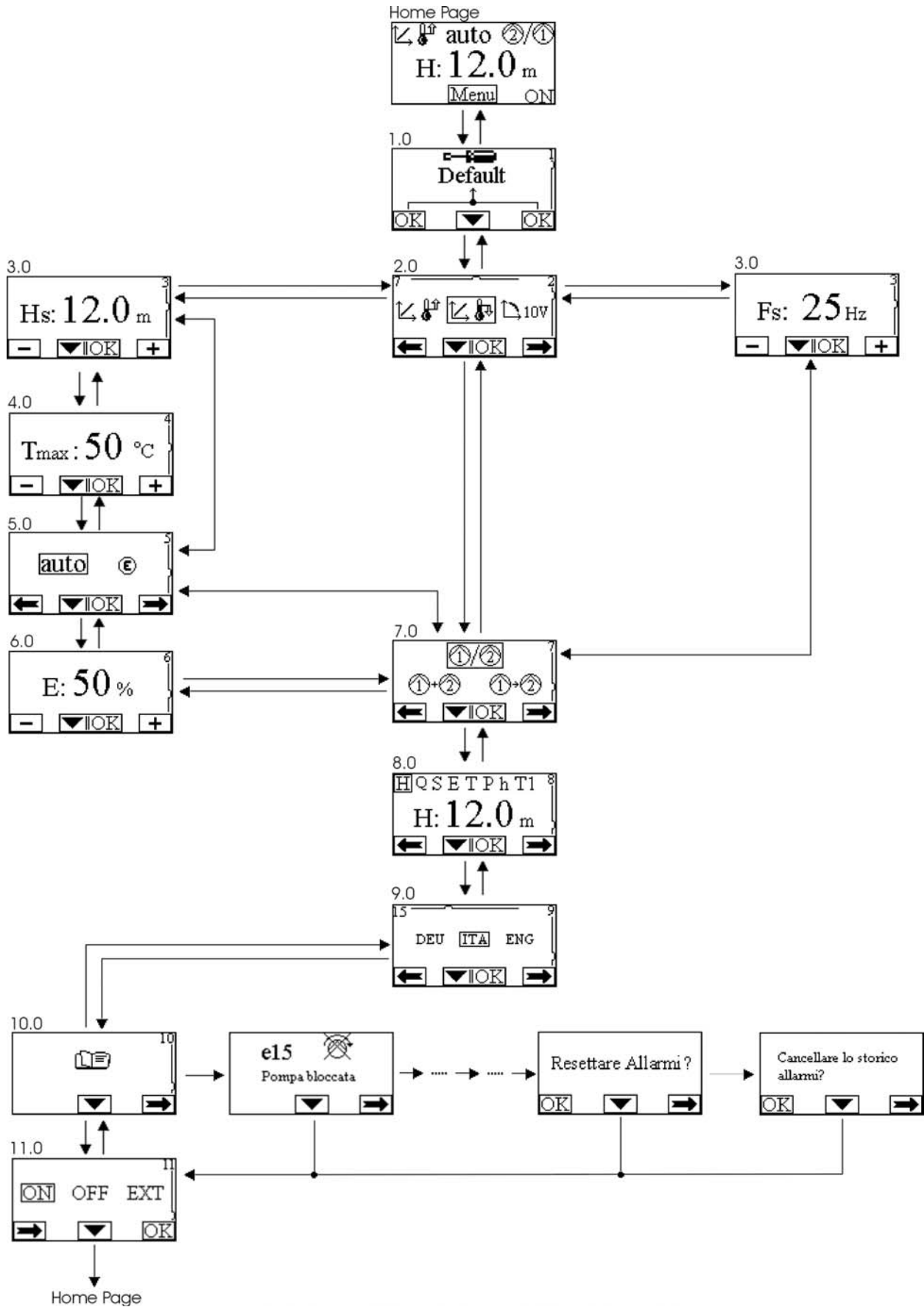
Figura 8: Menù MCE/C
