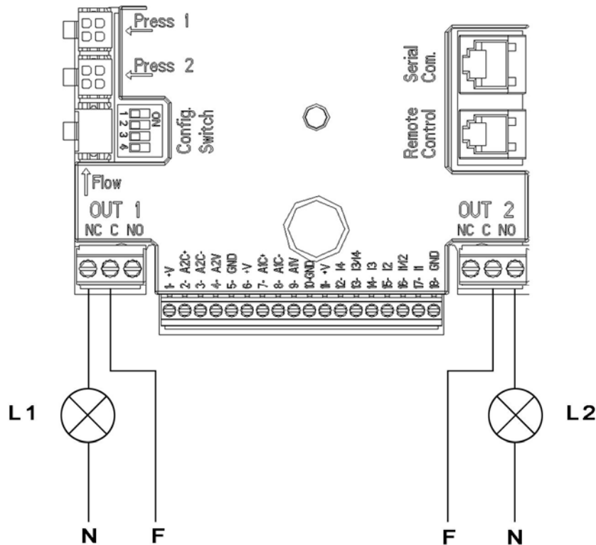
6.ábra: Digitális kimenetek bekötésére vonatkozó példa
