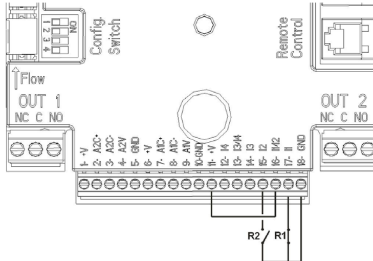
Фиг. 4: Пример за свързване на цифрови входове
