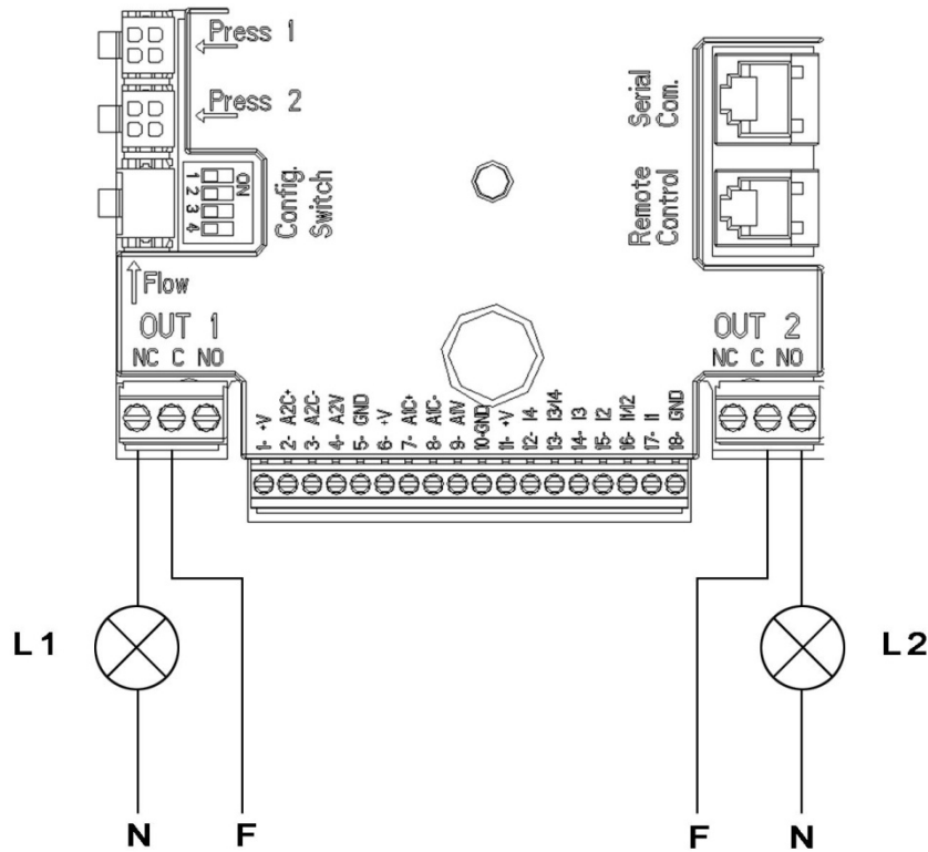
Фиг. 6: Пример за свързване на цифрови изходи
