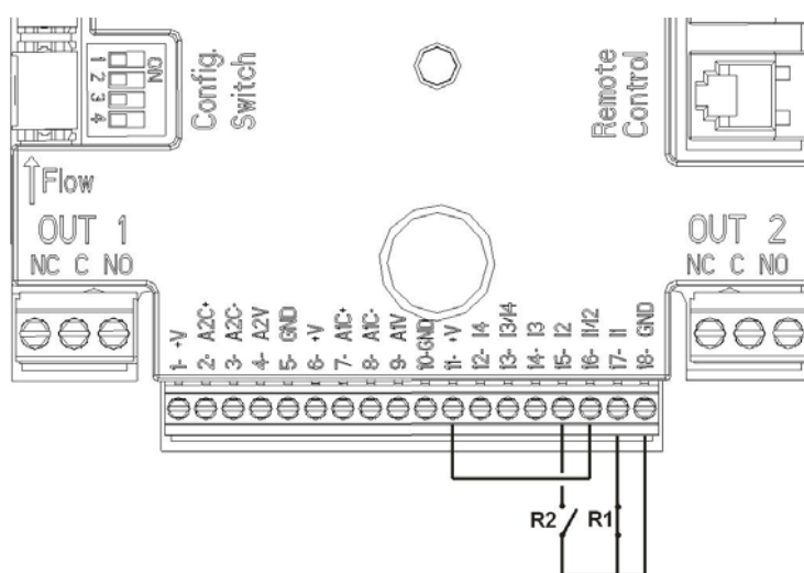
Abbildung 4: Anschlussbeispiel für Digitaleingänge
