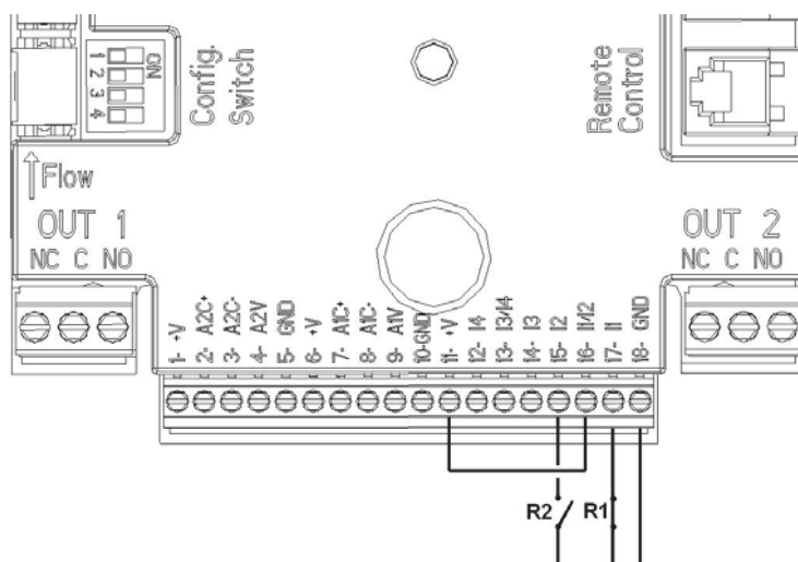
Figura 4: Esempio Collegamento Ingressi Digitali
