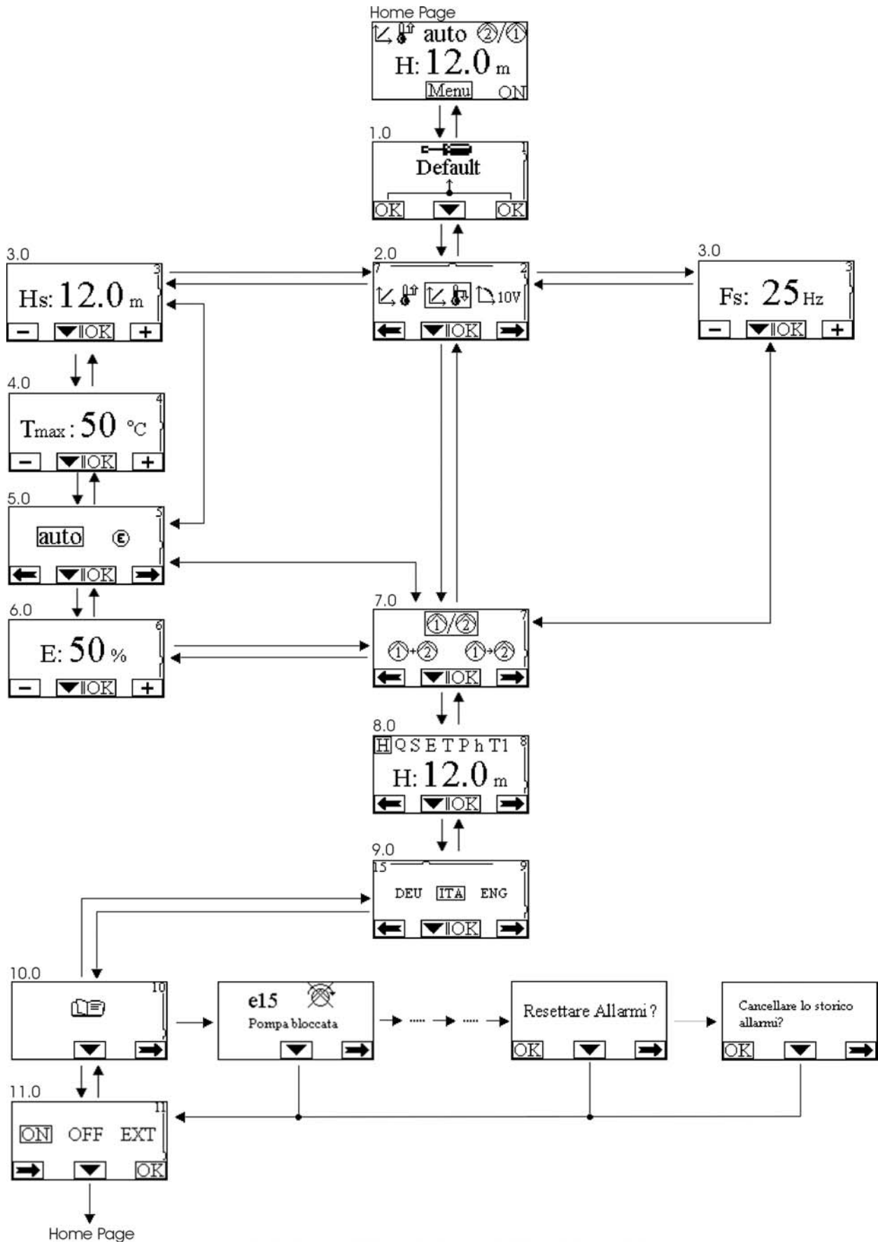
Afbeelding 8: Menu MCE/C
