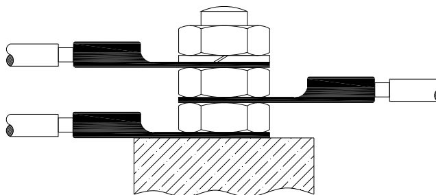
Figure 2 : Mise à la terre
