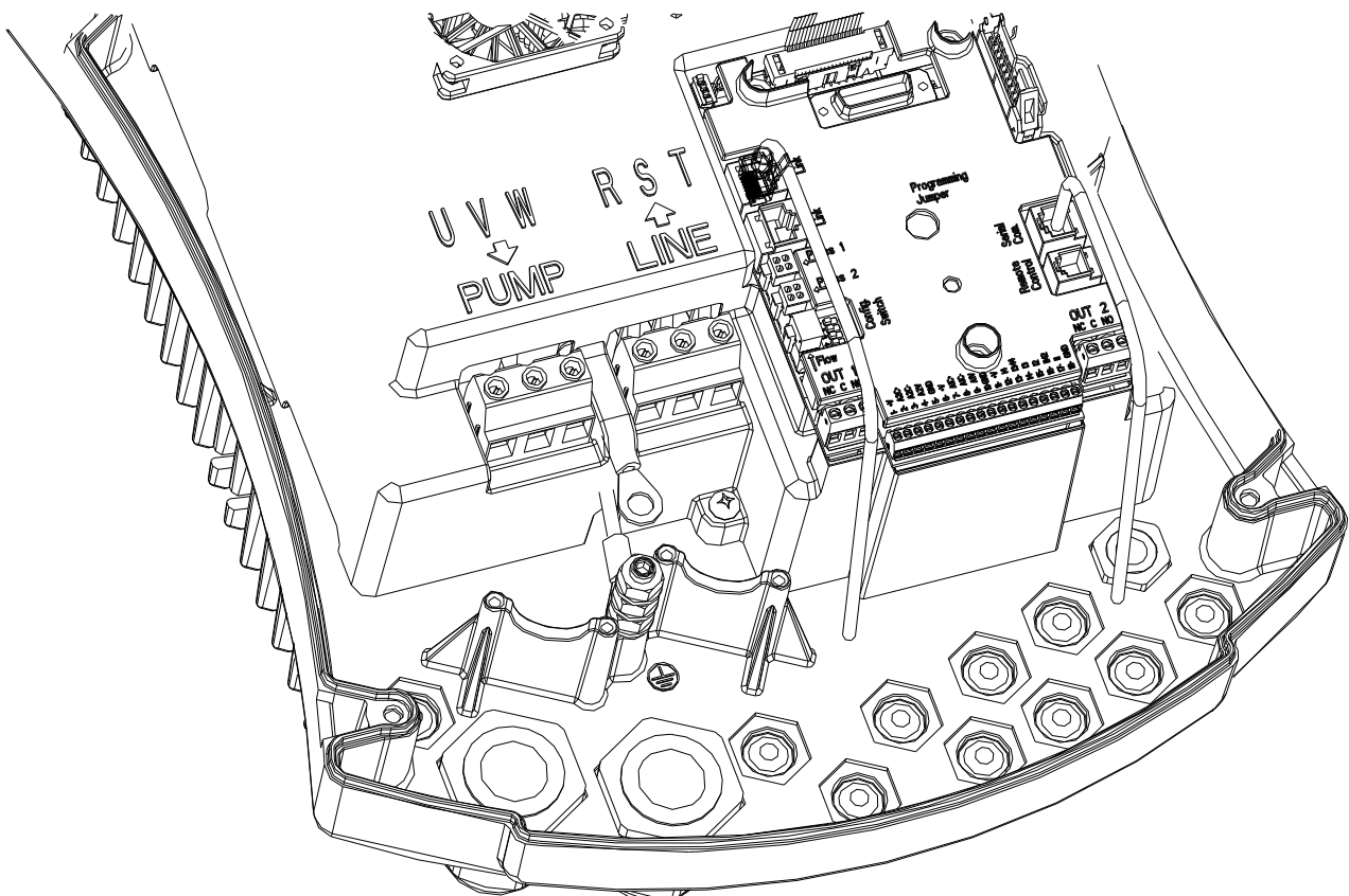
Σχήμα 1: Ηλεκτρική Συνδεσμολογία
