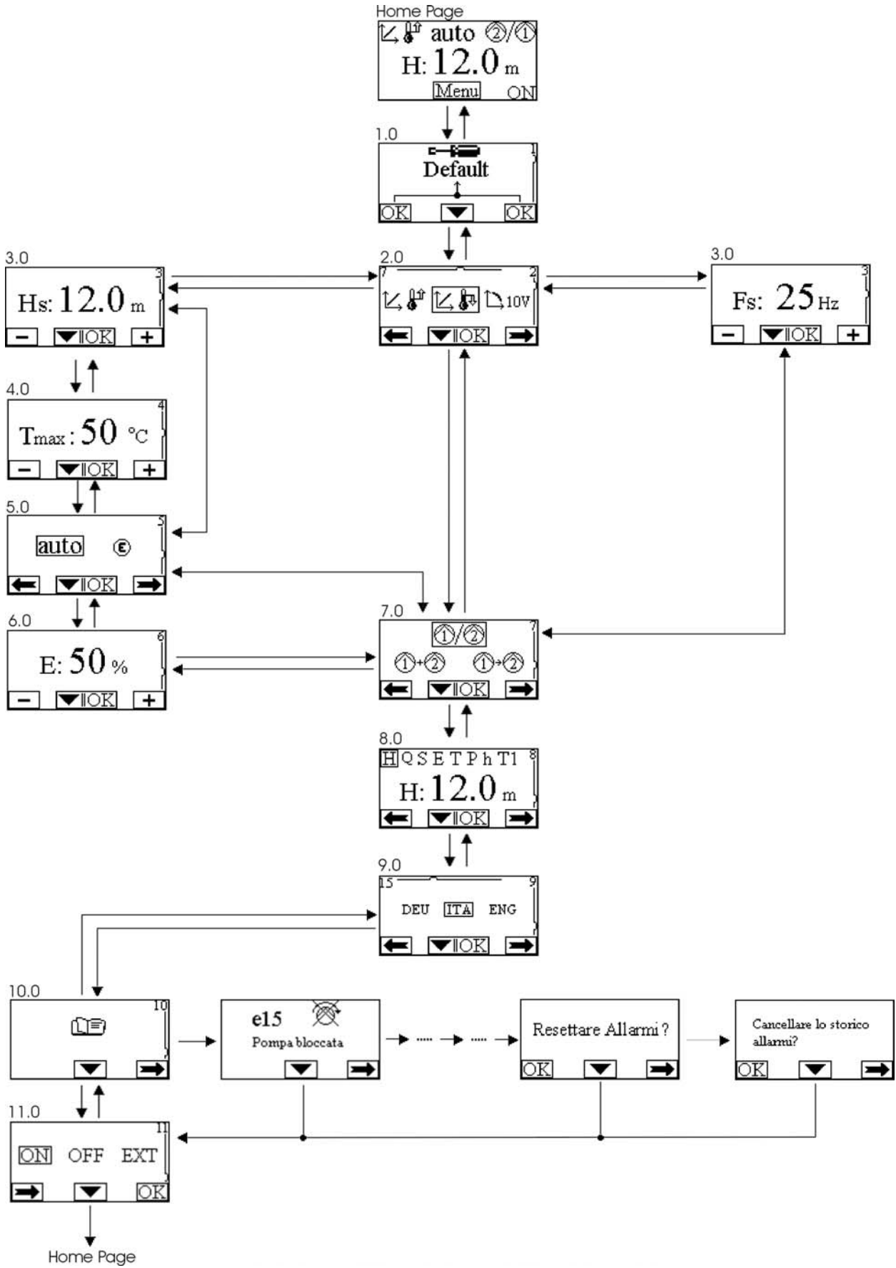
Σχήμα 8: Μενού MCE/C
