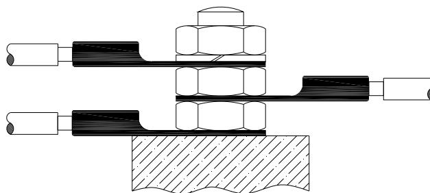
Фиг. 2: Заземяване
