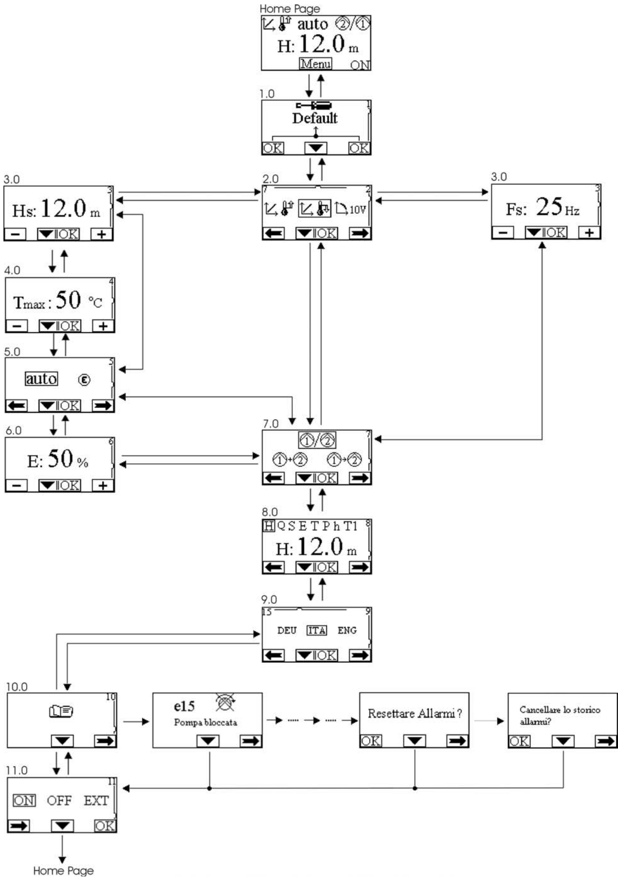
Abbildung 8: MCE/C-Menü
