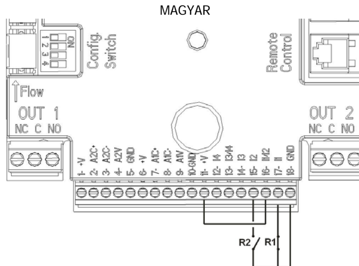
4. ábra: Példa digitális bemenetek bekötésére
