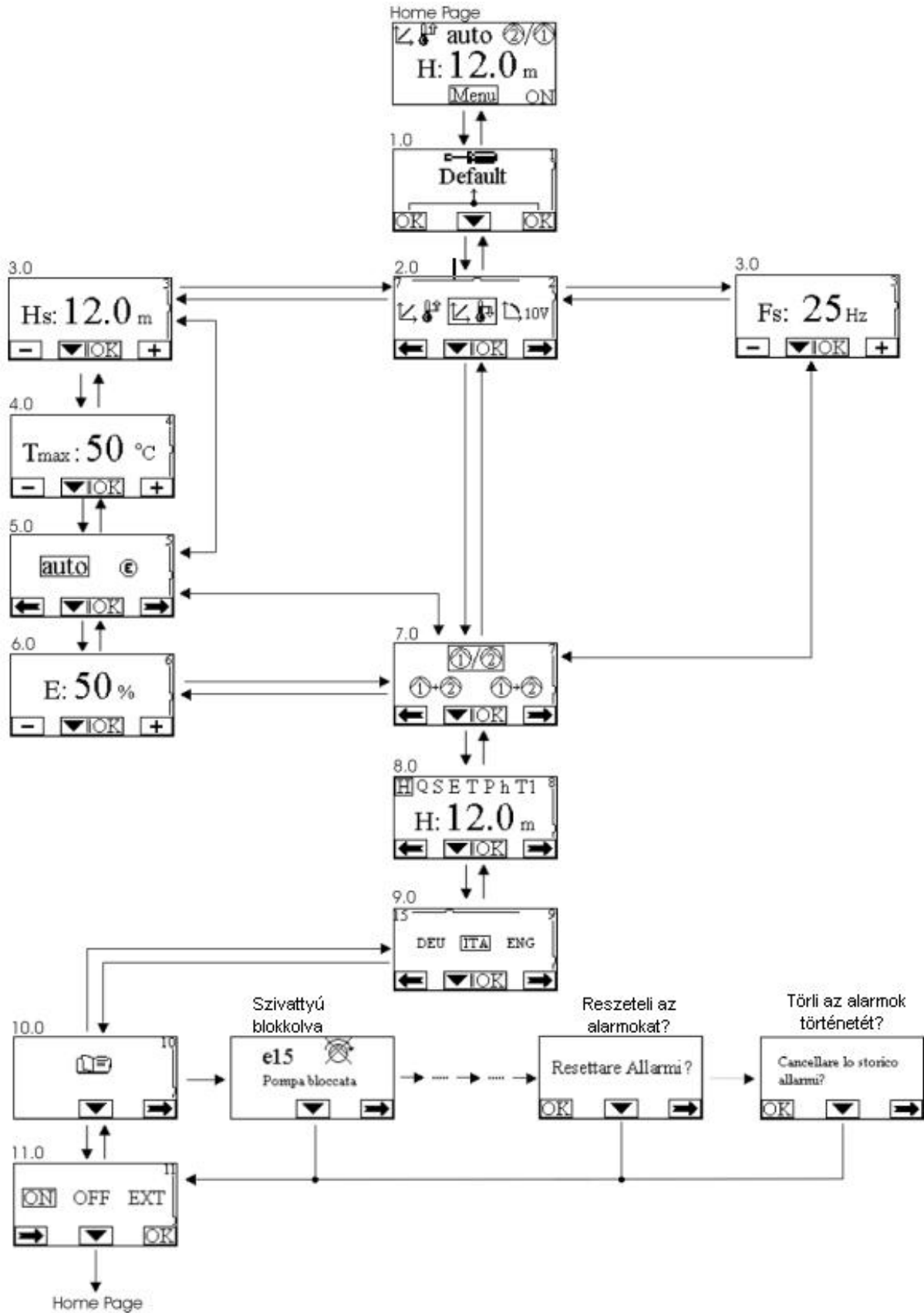
8..ábra: MCE/C menü
