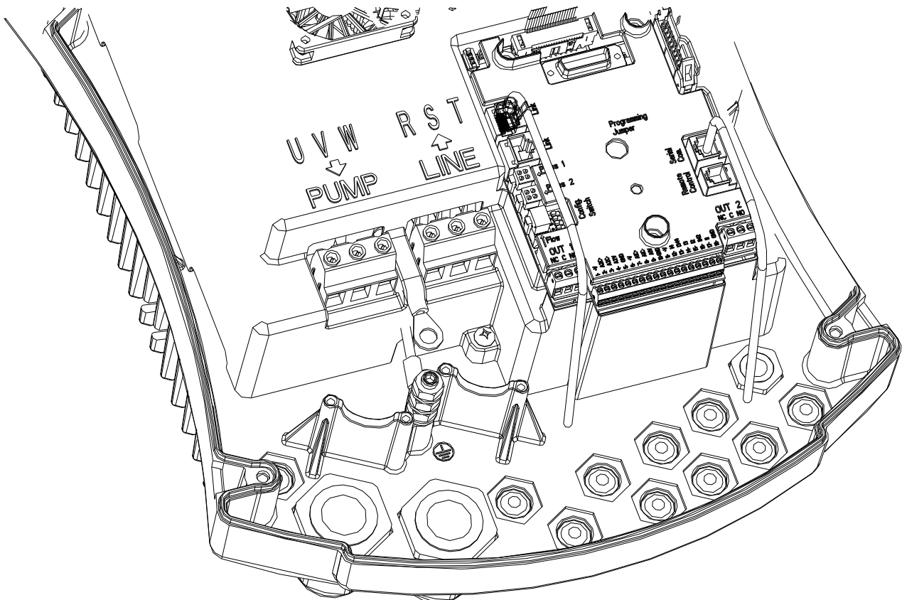
Фиг. 1: Електрически връзки
