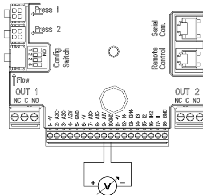
5. ábra: Analóg bemenetre vonatkozó bekötési példa
