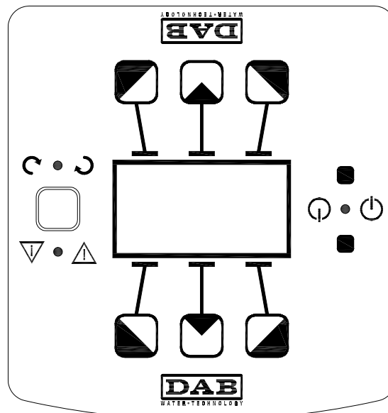
Abbildung 7: Steuerpaneel
