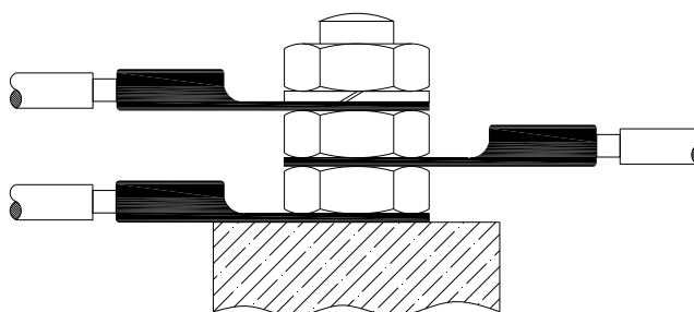
Figura 2: Împământare
