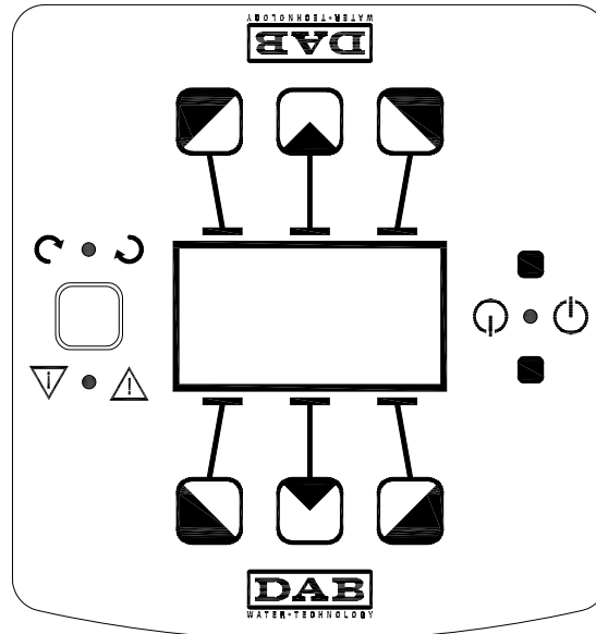
Slika 7: Kontrolna plošča
