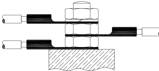
Resim 2: Toprak bağlantısı
