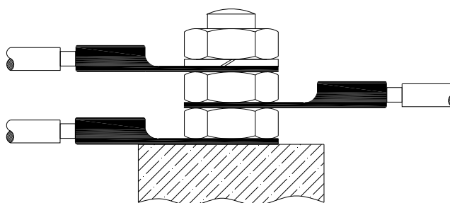
Σχήμα 2: Σύνδεση Γείωσης
