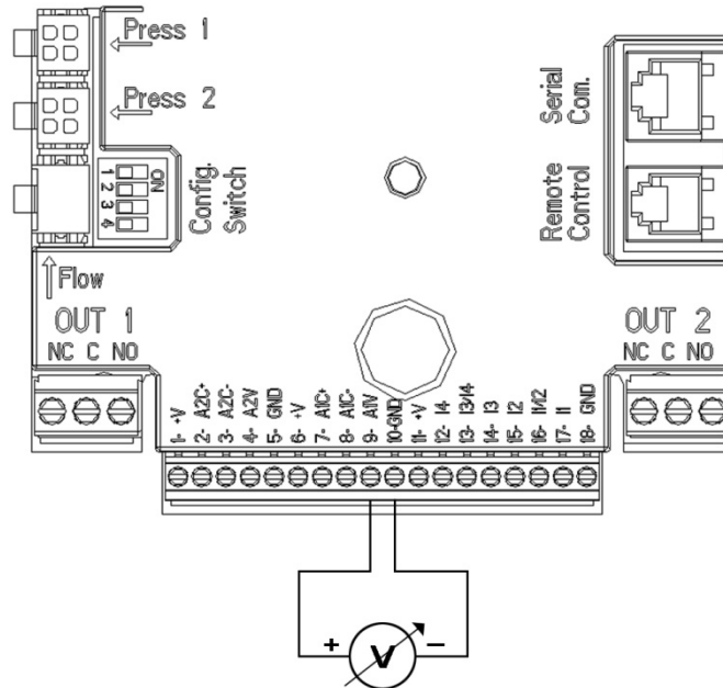
Фиг. 5: Пример на свързване на аналогов вход
