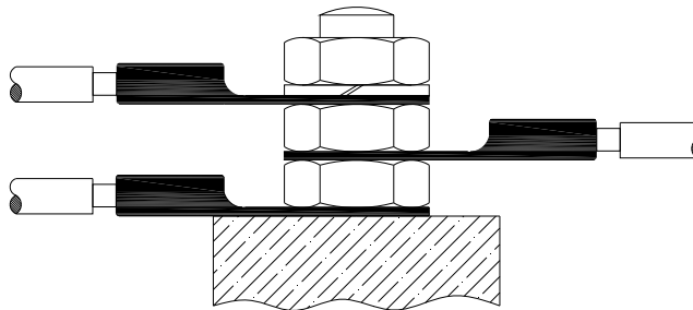
2.ábra: A védőföldelés bekötése
