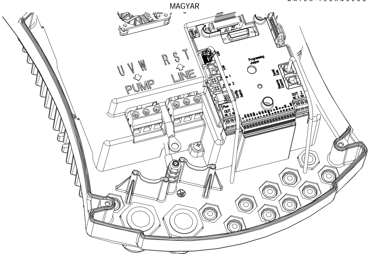
1. ábra: Elektromos bekötések
