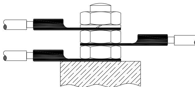
Abbildung 2: Erdungsanschluss
