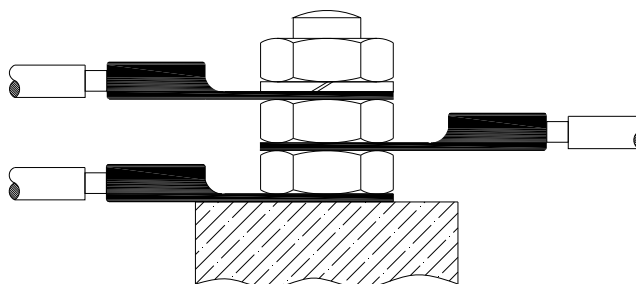
Figura 2: Conexión de tierra
